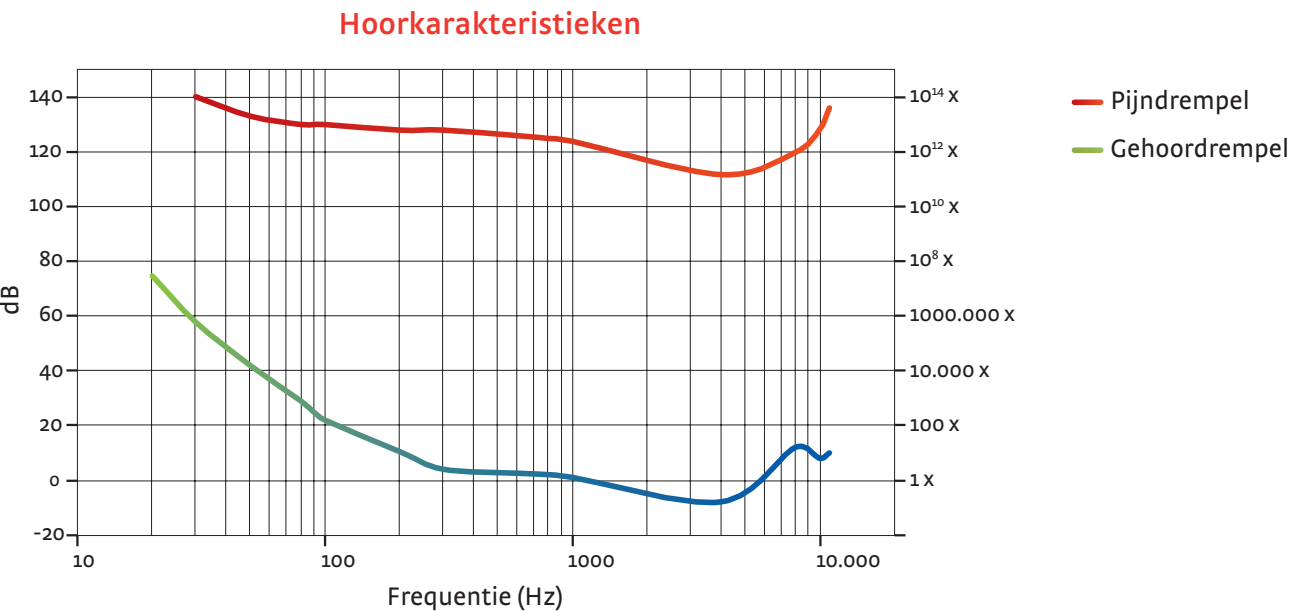
Figuur: Een audiogram waar de geluidsdrempel en de pijngrens zijn uitgezet tegen de frequentie voor de gemiddelde mens. Links staan dB's en rechts de factor die daar bij hoort
